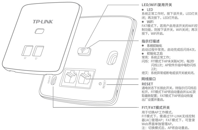
正面示意图
